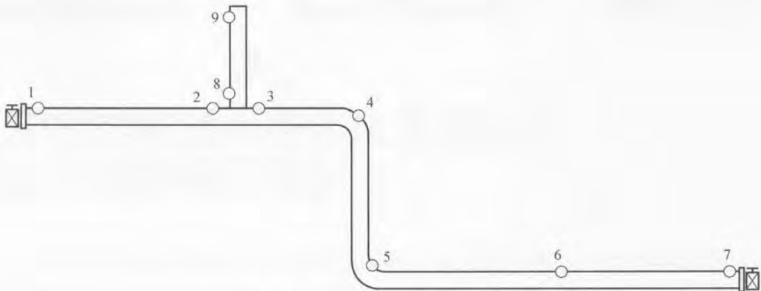
图 B.5 管道传感器布置示意图
